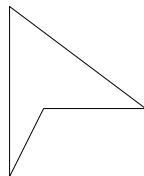
Рис. 4.13. Невыпуклый четырехугольник.
