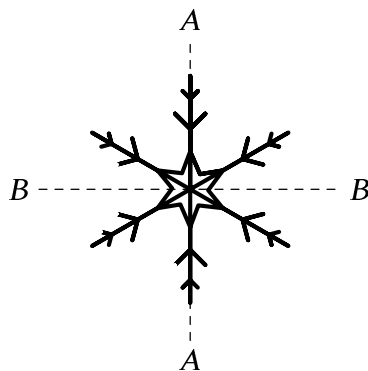
Рис. 4.28. Симметрии снежинки.
