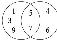
Рис. 4.8. Пересекающиеся множества.
